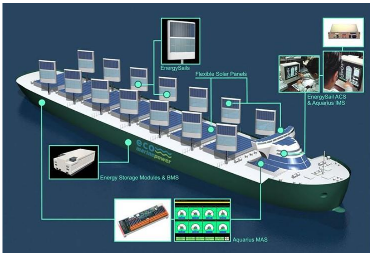
Figura 24: Primer buque de mercancías diseñado para captar energía eólica y solar
