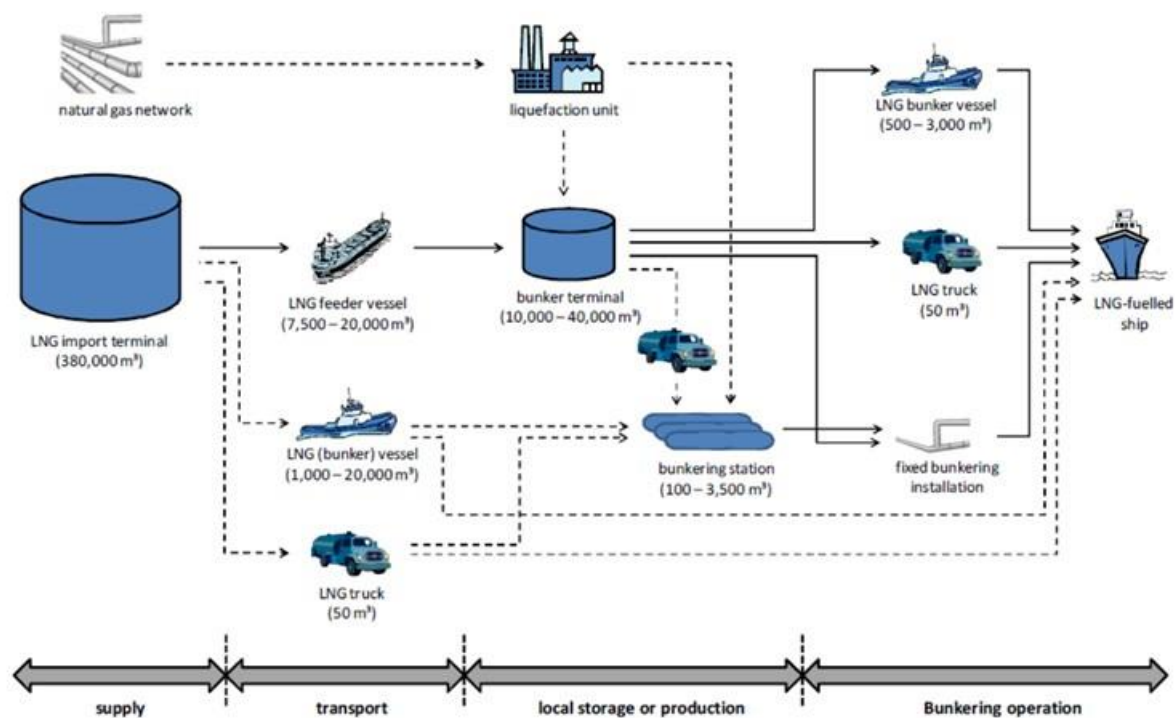
Figura 10: Representación esquemática de prácticas de aprovisionamiento de GNL
