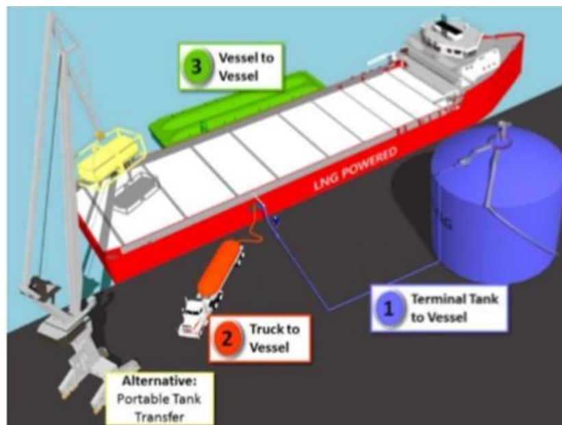
Figura 27: Esquema de transferencia de GNL "Camión – Buque" y "Tanque – Buque"
