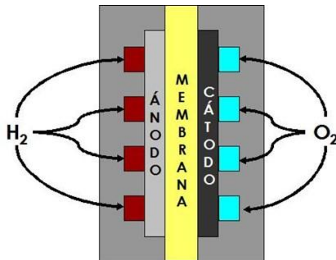
Figura B: Alimentación independiente de reactantes a cada electrodo a través de los canales de las placas de suministro.
