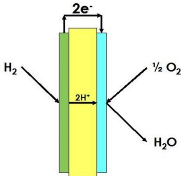
Figura A: Esquema de funcionamiento de una pila de combustible de hidrógeno.
